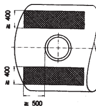
Doppelter Laufsteg
